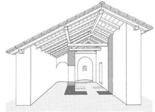
Рис. 1.68. Интерьер двухапсидного храма. Реконструкция. Вид с северо-запада. Fig. 1.68. Interior of the church, axonometric reconstruction, looking northwest.
