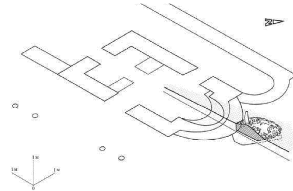
Рис. 1.62. Начальный этап освоения вершины холма Тузлук. Реконструкция. Вид с востока. Fig. 1.62. First stage of the cultural activity at the top of the Tuzluk hill, axonometric reconstruction, looking west.
