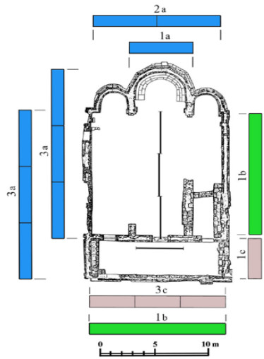
Рис. 1. План Эски-Керменской базилики с числовыми пропорциями (на основе плана 1930 г. [11, с. 217, рис. 56])
