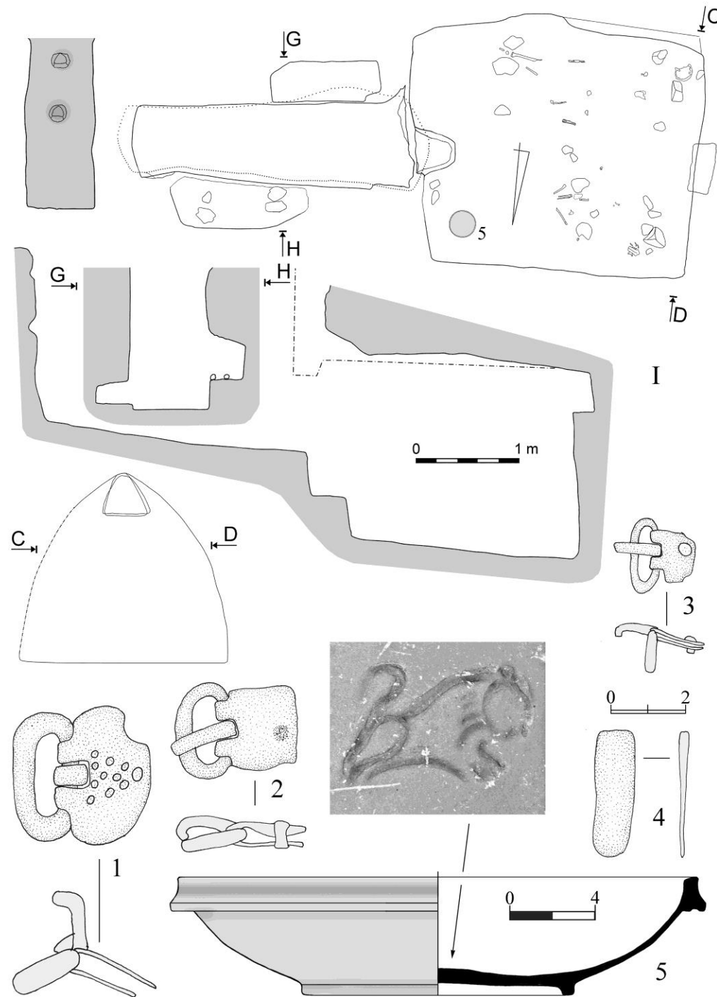
Рис. 10. Мангуп, могильник Алмалык- Дере. Склеп 188/2008. I – план склепа, разрезы к плану и фасировка тыльного борта дромоса; 1-5 – находки из склепа. [по Maçzyńska и др., 2016, Taf. 362; 365, 1,2,8; 366, 1,2]
