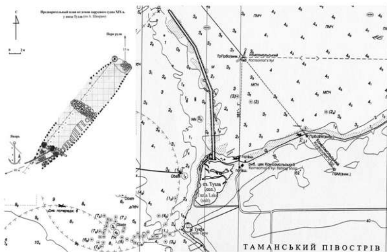
Рис. 1 Карта южной части Керченского пролива (акватория мыса Тузла). План остатков парусного судна XIX в.
