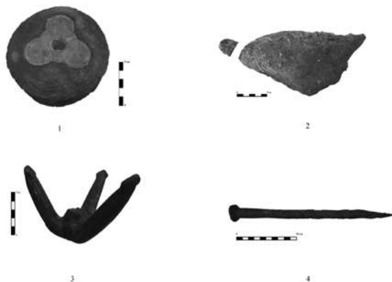
Рис.2 Детали оснастки судна. 1 – шкив блока, 2 – балластный камень, 3 – такелажная кошка (рым сломан), 4 – корабельный гвоздь.
